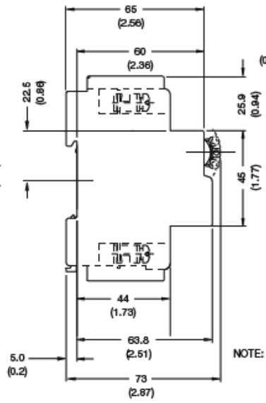
DIN RAIL MOUNT
